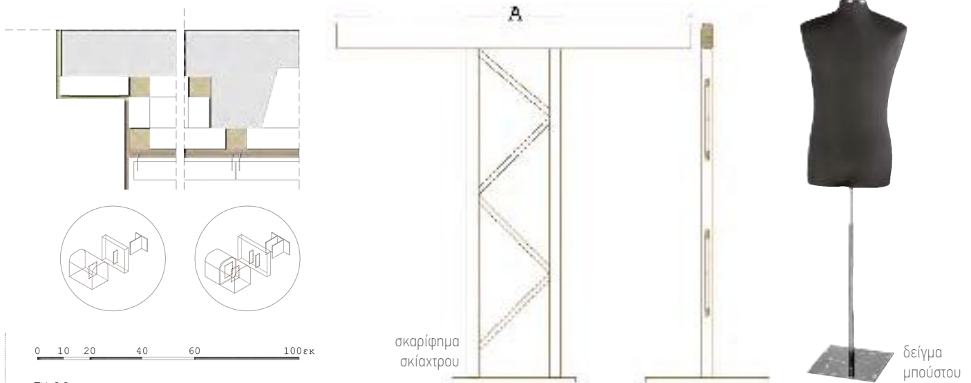
ΕΝΔΕΙΚΤΙΚΗ ΛΕΠΤΟΜΕΡΕΙΑ ΔΟΚΟΥ ΚΡΕΜΑΣΗΣ Ikat ΕΝΤΟΣ ΠΡΟΘΗΚΗΣ
